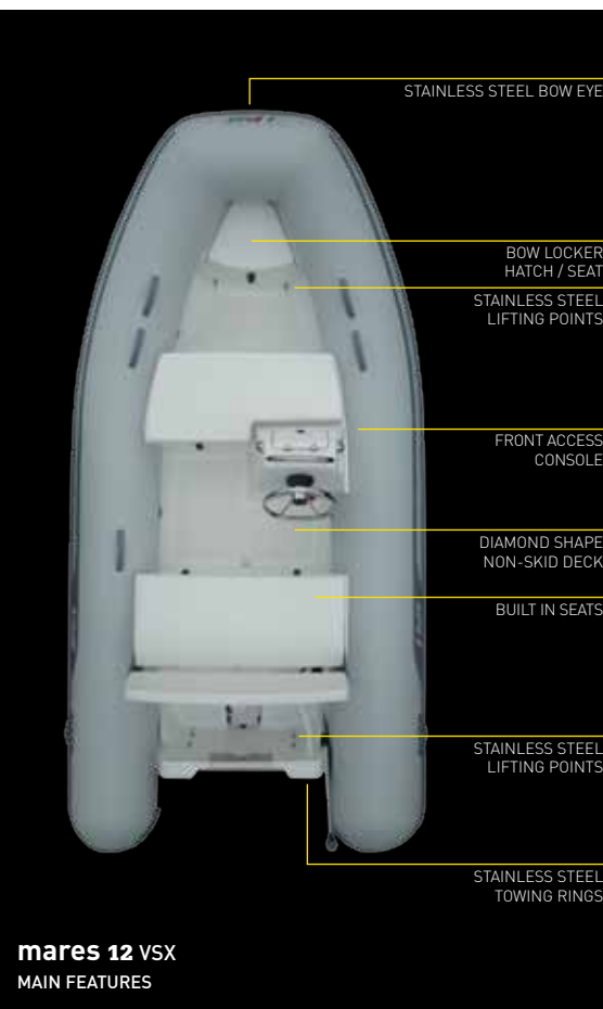
mares 12 VSX
