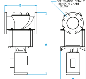
HSE DIMENSIONS
