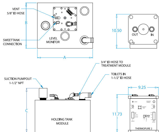
TP-210 DIMENSIONS
