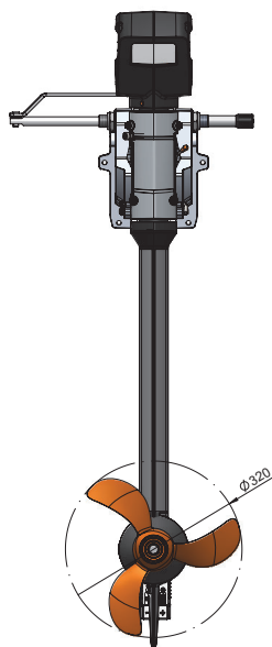
Propeller B 12,5 x 17 HSP
