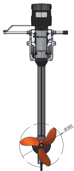
Propeller B 12 x 10,5 WDR
