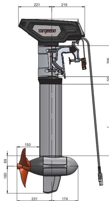
Propeller B 12,5 x 17 HSP
