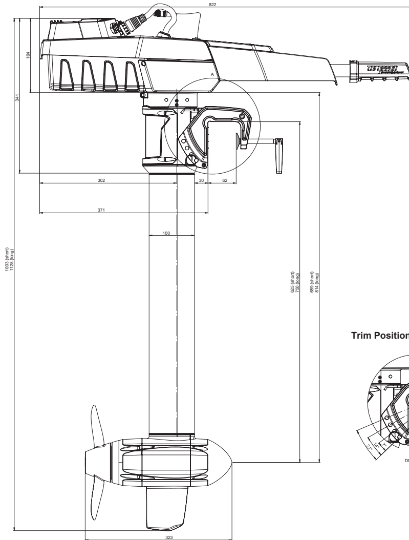
Side View / Seitenansicht
