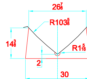
TRANSVERSAL SECTION "B" SECCION TRANSVERSAL "B"
