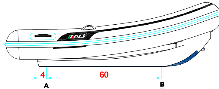
LONGITUDINAL PROFILE PERFIL LONGITUDINAL
