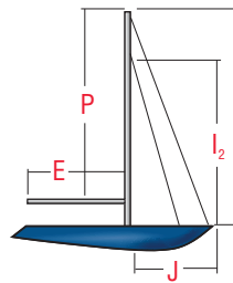
Rig Dimensions
